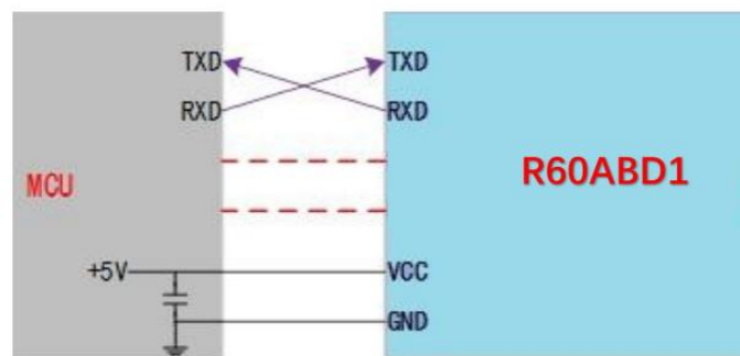
雷达模块与外设连线示意图
