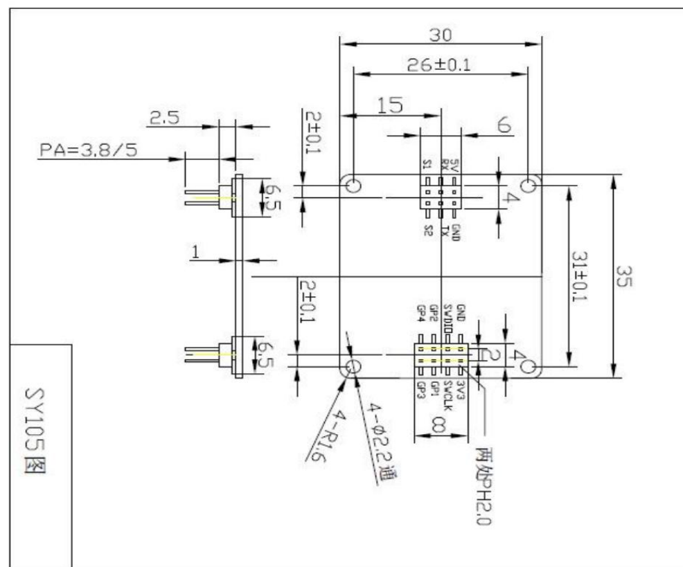
图 2: 雷达模块结构示意图
