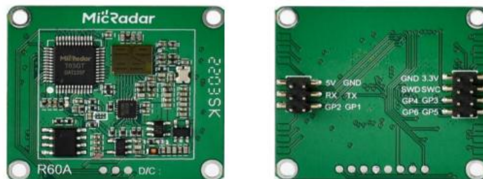
图 1：雷达正反面照片
